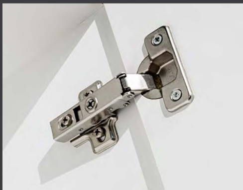
Zawiasy z cichym domykaniem, regulowane w trzech płaszczyznach.
