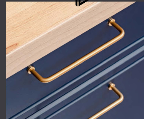
Blaty o grubości 38 mm w technologii postforming (promień zaoblenia krawędzi R=3 mm).
